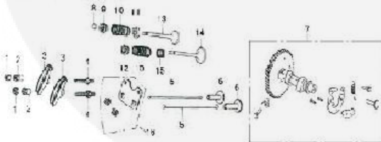
Camshaft
